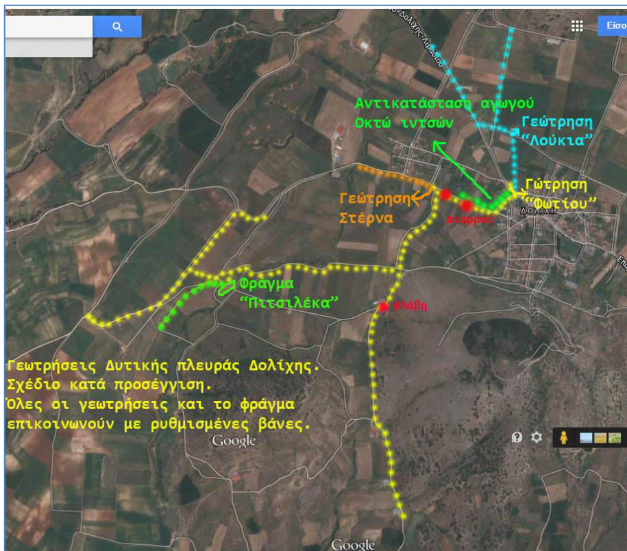
Εικόνα 6: Αποτύπωση γεωτρήσεων και αγωγών άρδευσης δυτικής πλευράς
