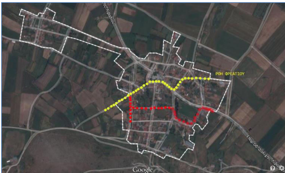
Εικόνα 7: Οι αγωγοί μετακίνησης όμβριων υδάτων
